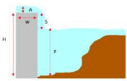
Variables para obstáculos de salto vertical
