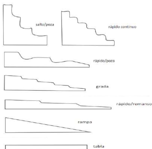
Figura 34.- Tipo de estructuras longitudinales
