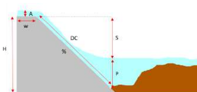
Figura 11.-Variables para obstáculos tipo paso sobre paramento
