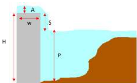
Figura 9.-Variables para obstáculos de salto vertical
