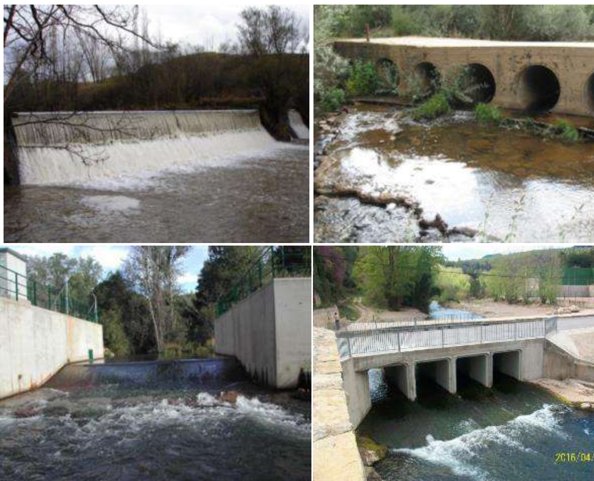
Figura 8: Ejemplo de obstáculos (de arriba a abajo y de izquierda a derecha): salto vertical, paso entubado mixto, pa sobre paramentos, obstáculo mixto
