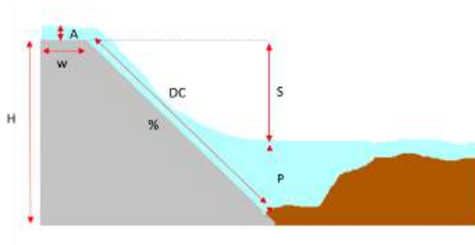
Variables para obstáculos tipo paso sobre paramento
